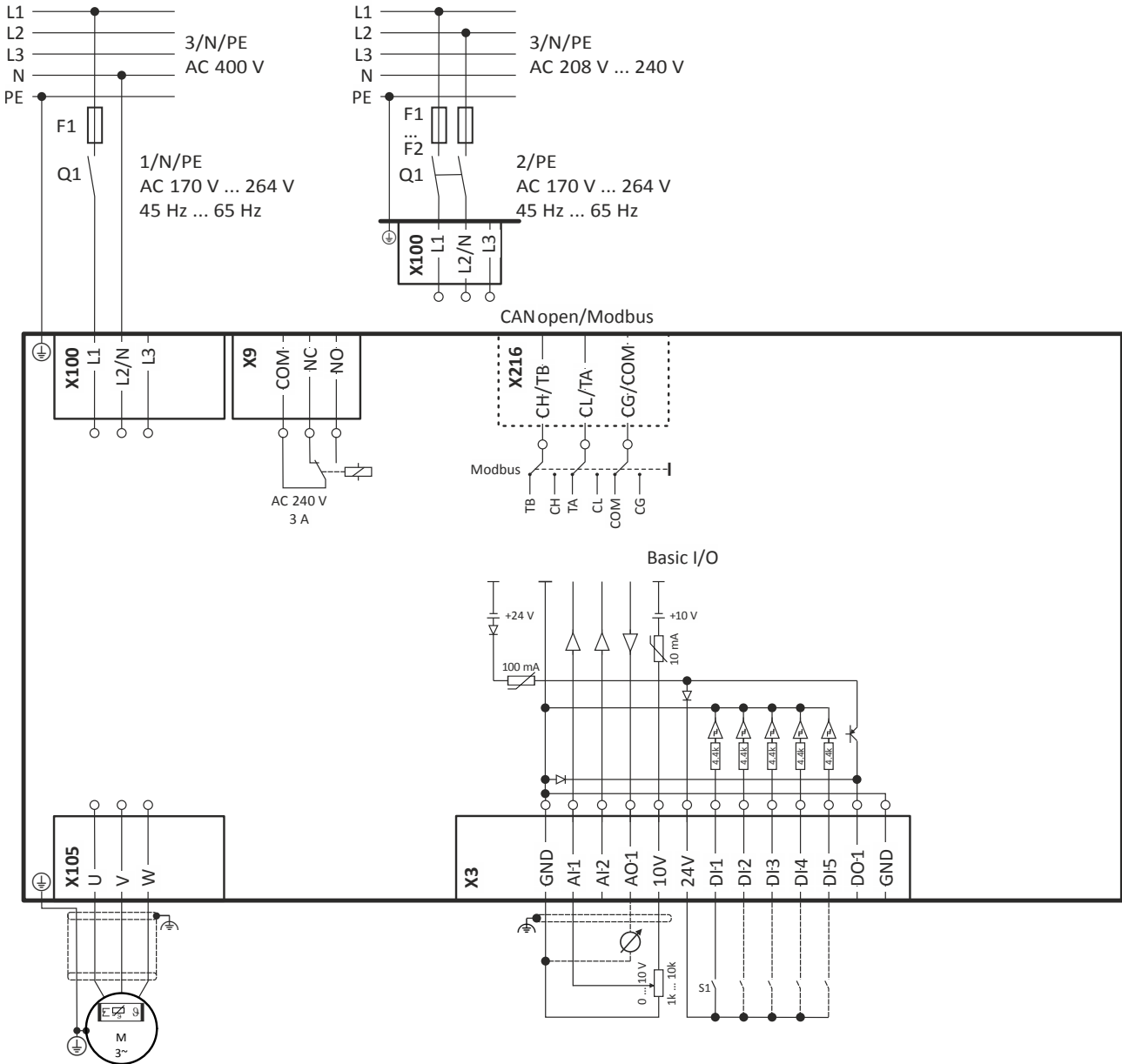
Fig. 4: Wiring example
